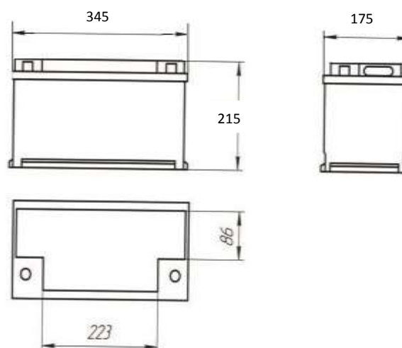
Габариты тип ГОСТ
